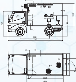
(Bản vẽ Model ATV - XXN - 2021DD2)
