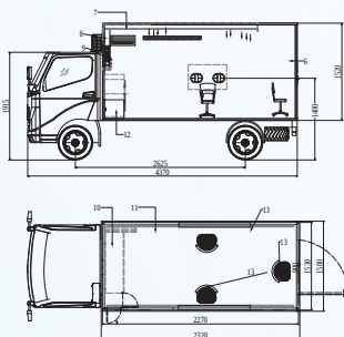
(Bản vẽ Model ATV - XXN - 2021DD3)
